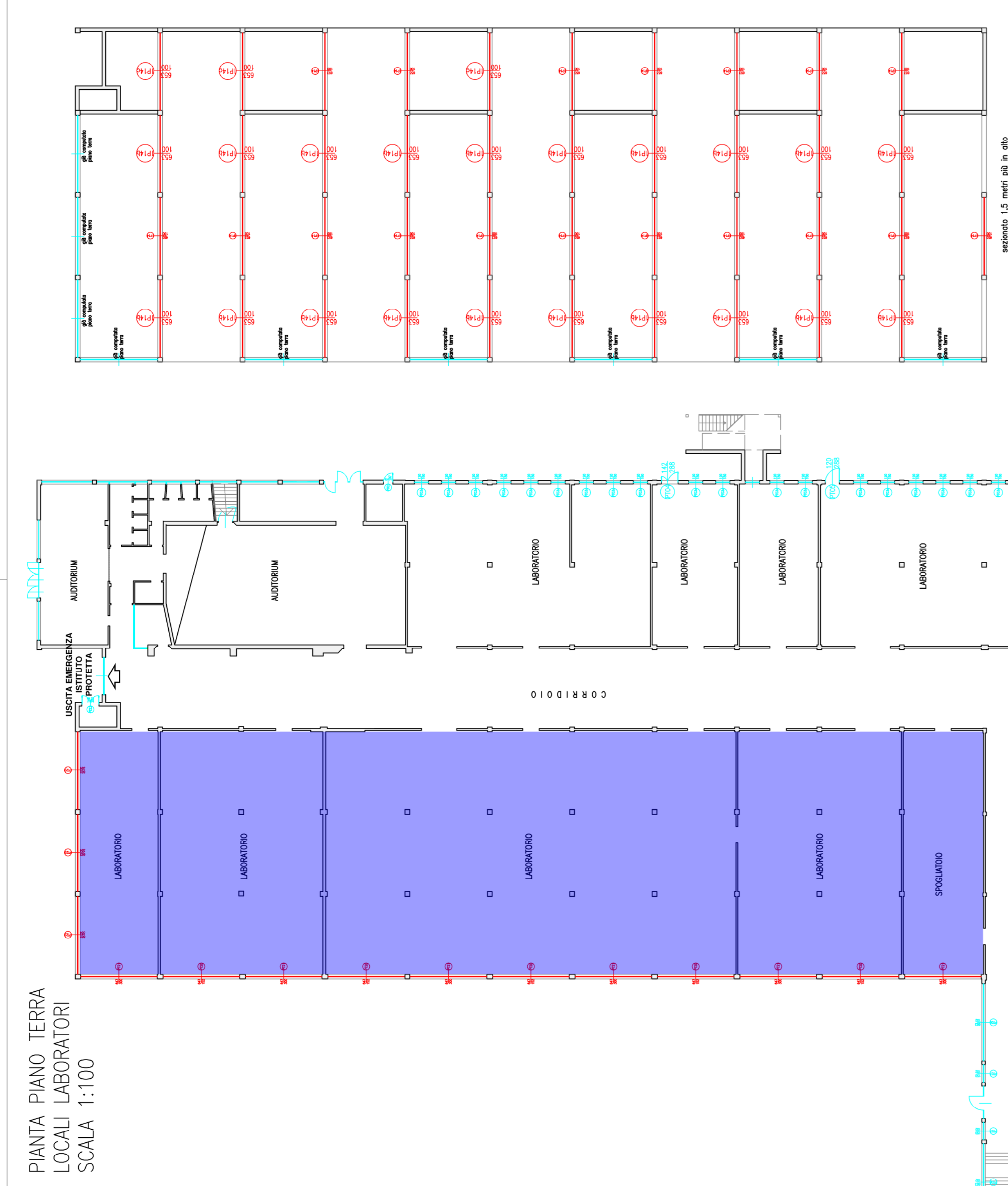
PIANTA DELLA COPERTURA LOCALI LABORATORI SCALA 1:100
